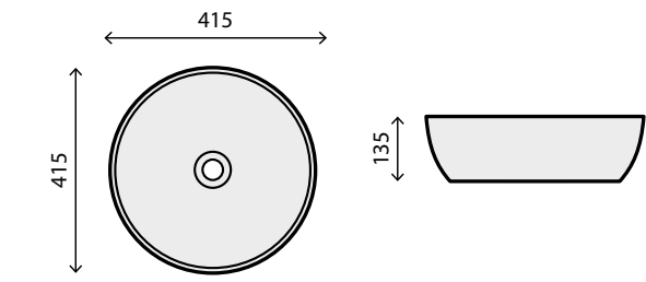
RS428WSIL S150/225 Dim.: Ø 41,5 x 13,5 cm Pack: 7 kg / 0,029 m³
