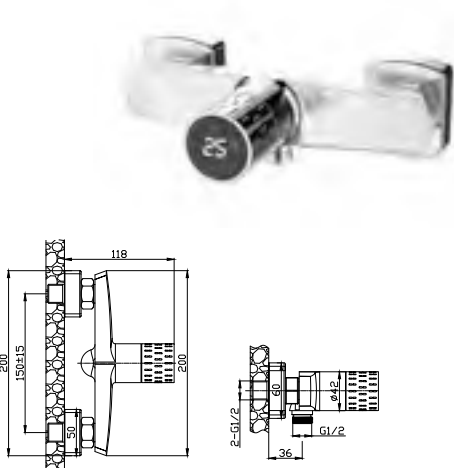
MONOCOMANDO DUCHE TAI50/225 Ref.: RTD28304BACR Pack: 4 kg / 0,008 m³ Single Lever / Mitiger / Mischbatterie / Monomando
