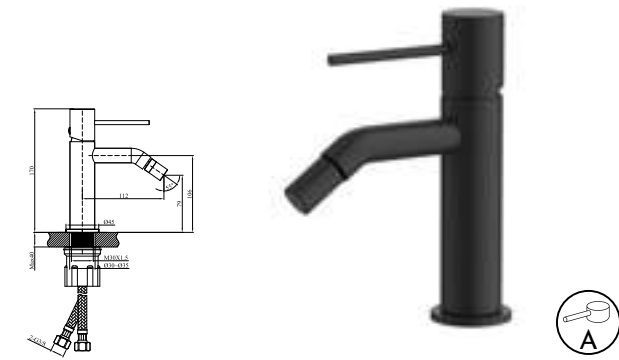
MONOCOMANDO BIDÉ TA80/120 Ref.: RT0392BIPRM Pack: 1,24 kg / 0,005 m³ Single Lever / Mitiger / Mischbatterie / Monomando
