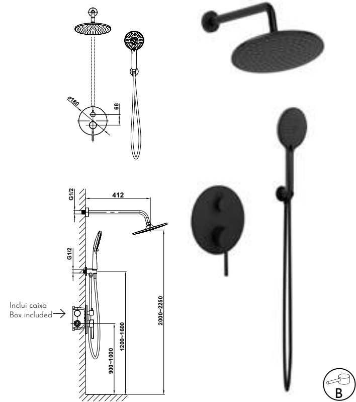
KIT DUCHE TA220/330 Ref.: RKE039PRM Pack: 6 kg / 0,09 m³ Single Lever / Mitiger / Mischbatterie / Monomando
