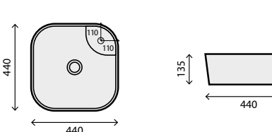
RS78202 S85/128 Dim.: 44 x 44 x 13,5 cm Pack: 9,5kg / 0,033m³
