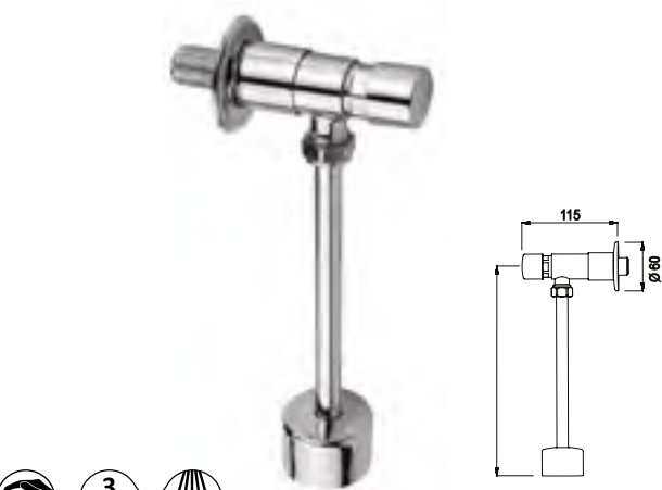
FLUXÓMETRO URINOL Ref.: RT14300031 Pack: 1,5 kg / 0,004 m³ Urinal / Urinoir / Urinal / Urinario
