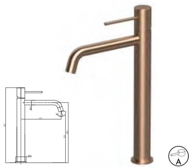
MONOCOMANDO LAV. TA110/165 Ref.: RT0393LAARSGM Pack: 2 kg / 0,009 m³ Single Lever / Mitiger / Mischbatterie / Monomando
