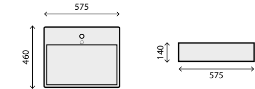
RS7669B S170/255 Dim.: 57,5 x 46 x 14 cm Pack: 16kg / 0,045m³
