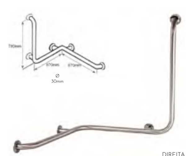
BARRA DE APOIO INOX ESCOVADO TA200/300
