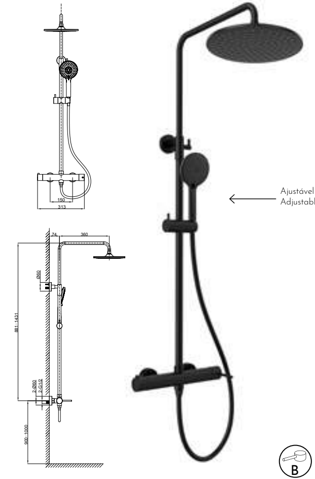
RAMPA DE CHUVEIRO TA250/375 Ref.: RRO39PRM Pack: 4,92 kg / 0,05 m³ Single Lever / Mitiger / Mischbatterie / Monomando
