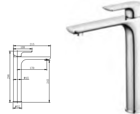
MONOCOMANDO LAV. TA160/240
