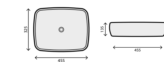
RS78105MCP S150/225 Dim.: 45,5 x 32,5 x 13,5 cm Pack: 7 kg / 0,025 m³
