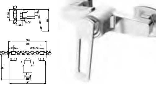
MONOCOMANDO DUCHE TA90/135
