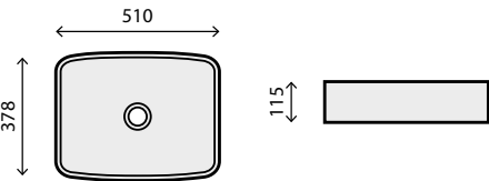
RS78535 S90/135 Dim.: 51 x 37,8 x 11,5 cm Pack: 11 kg / 0,028 m³
