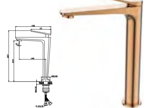
MONOCOMANDO LAV. ALTO TA130/195
