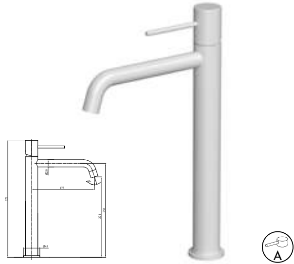
MONOCOMANDO LAV. TA90/135 Ref.: RT0393LAABRM Pack: 2 kg / 0,009 m³ Single Lever / Mitiger / Mischbatterie / Monomando
