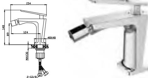
MONOCOMANDO BIDÉ TA80/120
