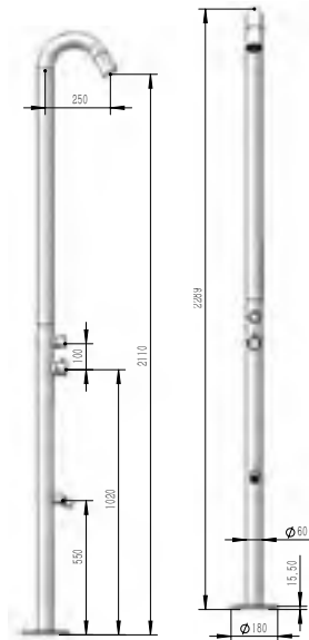
MONOCOMANDO INOX SPA1185/1778 Ref.: RCLML9002BL Pack: 17 kg / 0,12 m³ Single Lever / Mitiguer / Mischbatterie / Monomando
