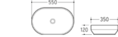
Válvula incluída / Drain included / Bonde incluse / Válvula incluida / Ventil enthalten RS6594CZESCMT S140/210 Dim.: 55 x 35 x 12 cm Pack: 6kg / 0,03m³
